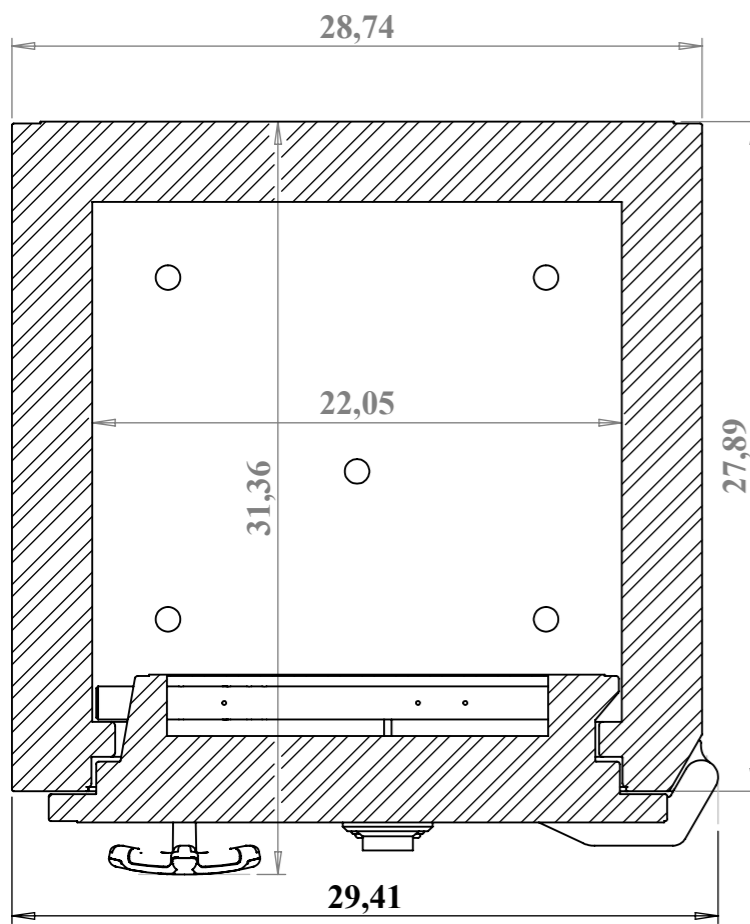
F-F (1 : 8)
