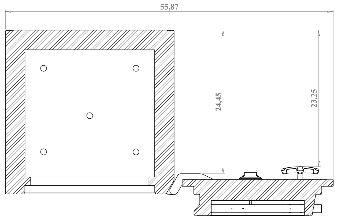
D-D (1 : 8)
