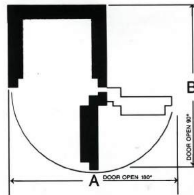
Door Swing Diagram
